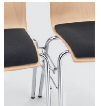
Modell 9011/S: mit Stapelsteg außen und Einhak-Reihenverbindung
